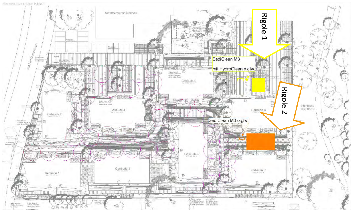
Abbildung 4 Positionierung der Rigolen
