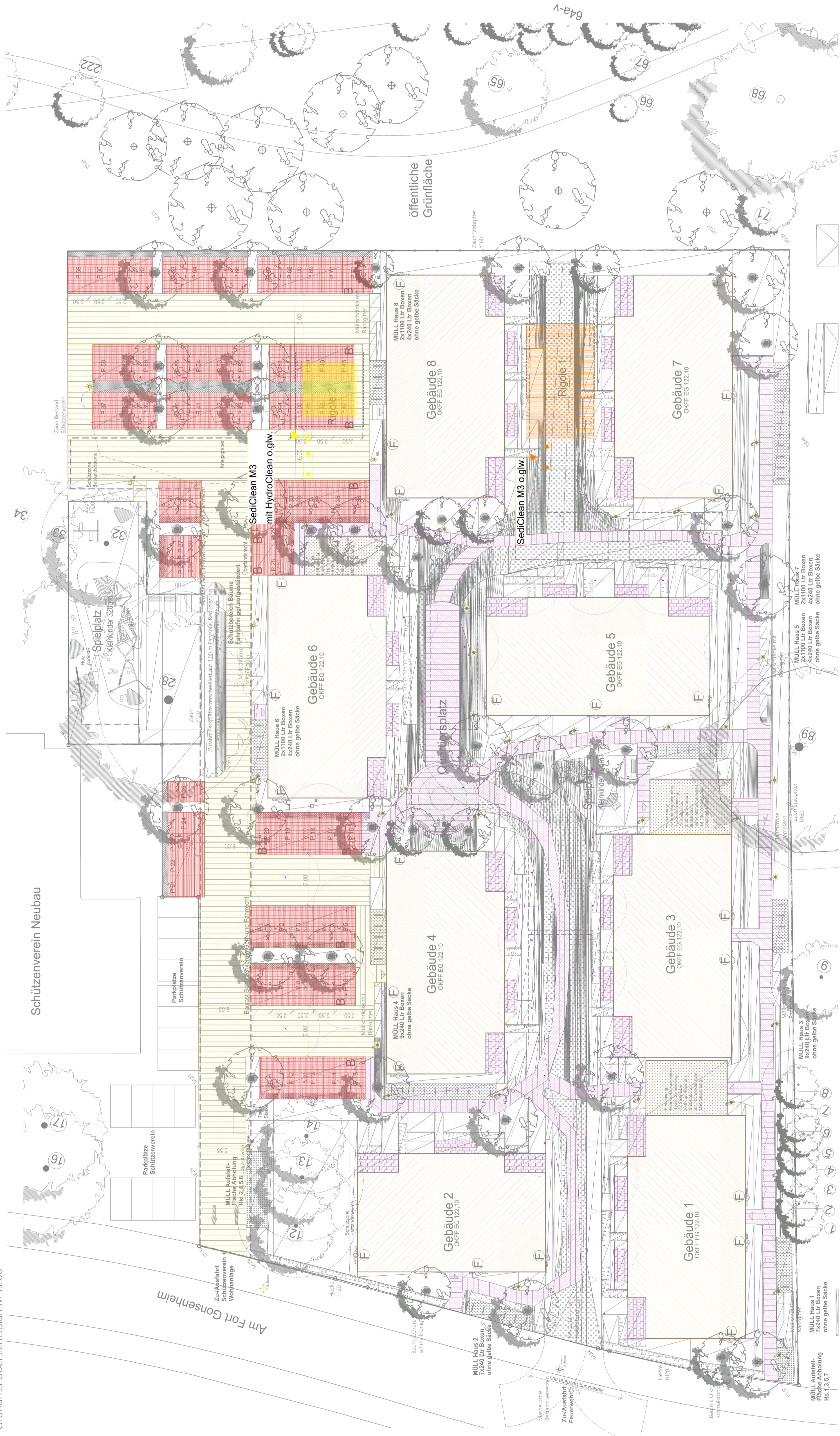
Grundriss Übersichtsplan M 1:200
